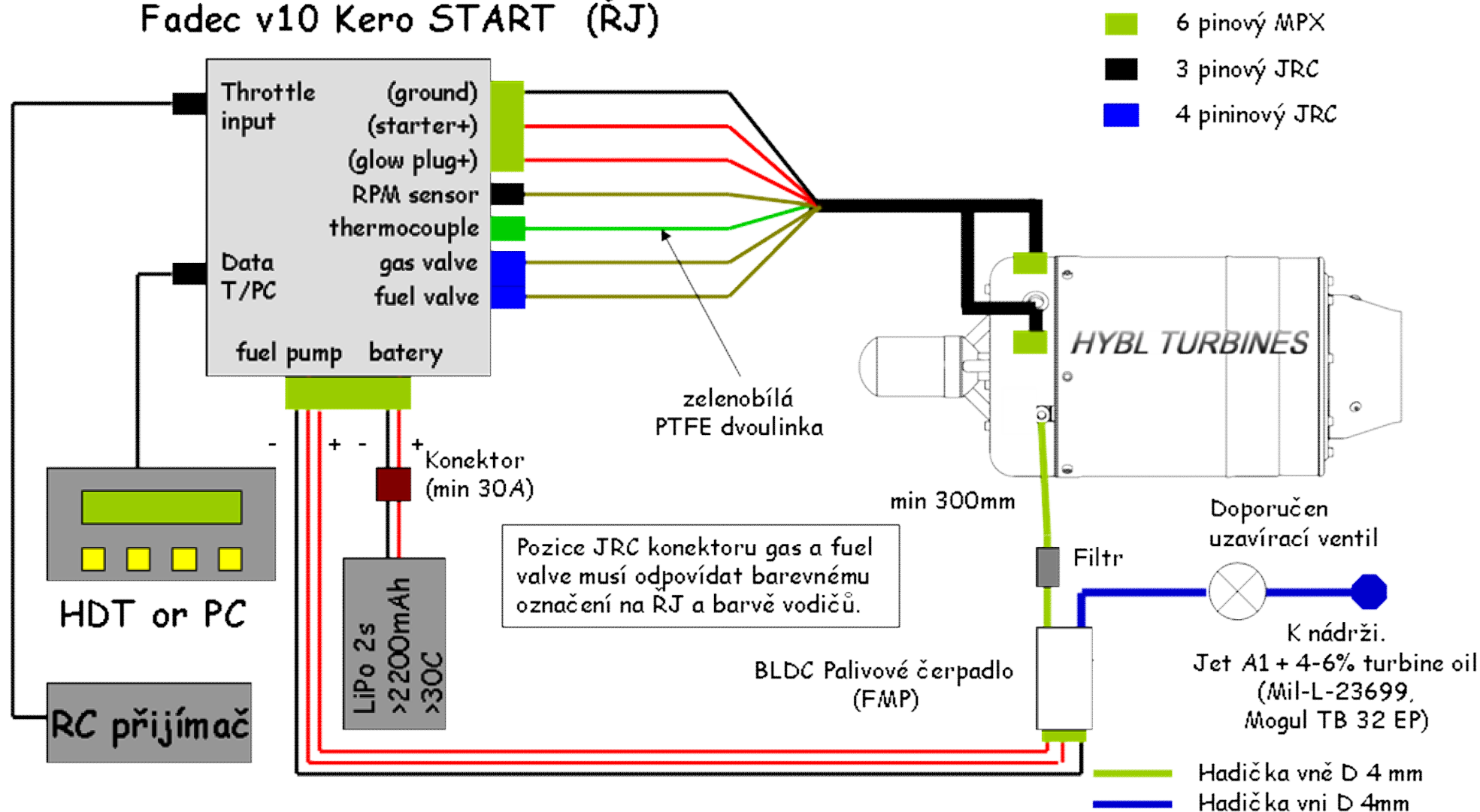
obr. 11 – schema zapojení palivové a elektrické instalace
