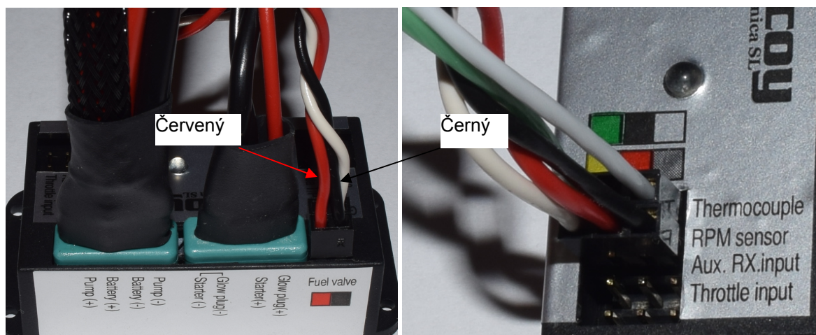
obr. 9 – zapojení kabelového svazku do ŘJ
