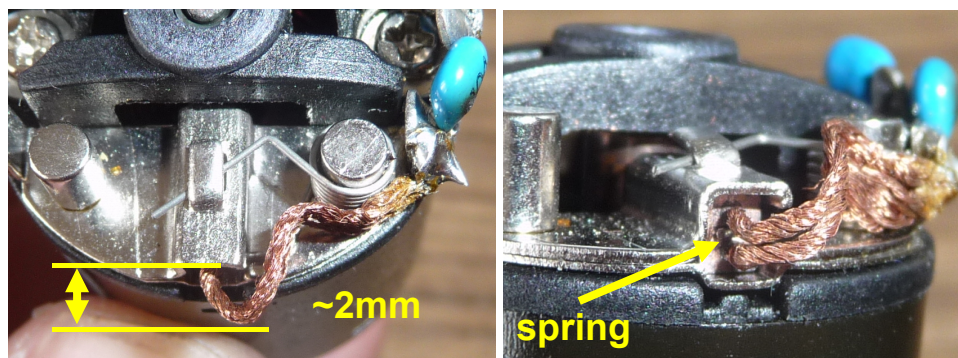
obr. 16 – natvarování přívodních vodičů k uhlíkům – vytvarovat oblouk – vodiče se nesmí dotýkat žádné části držáku uhlíku – opěrná pružinka v zárezu uhlíku a mezi vodiči
